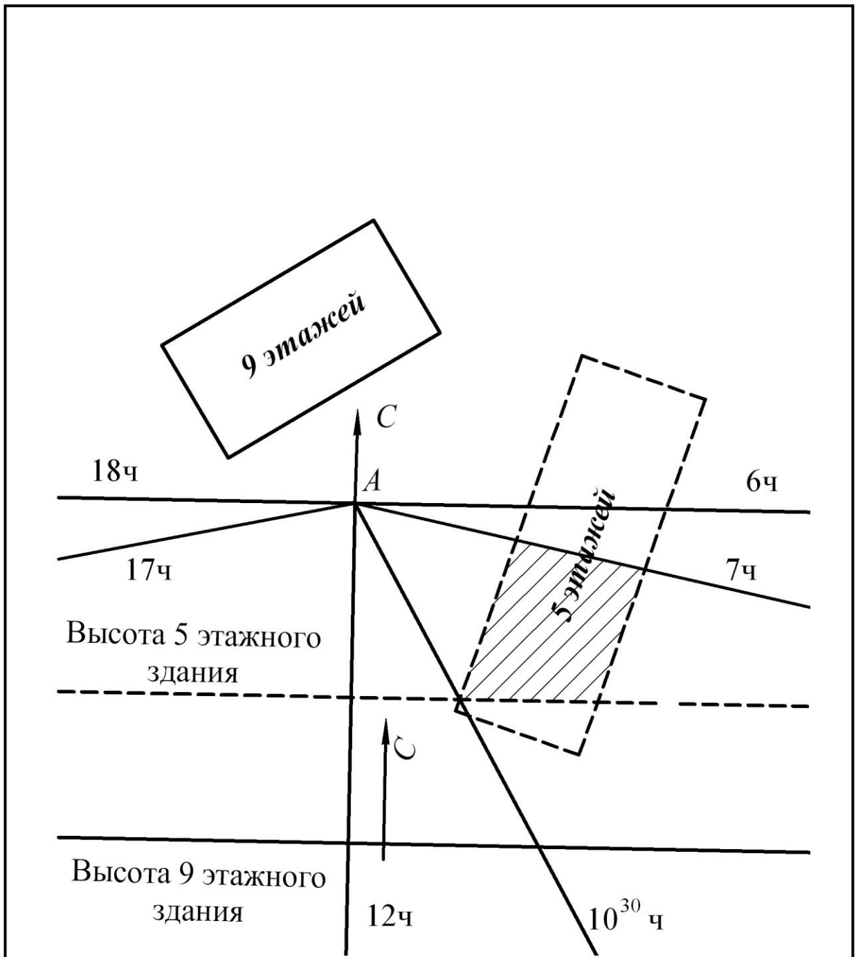
Рисунок 3.6 – Определение продолжительности инсоляции (М 1:500)
