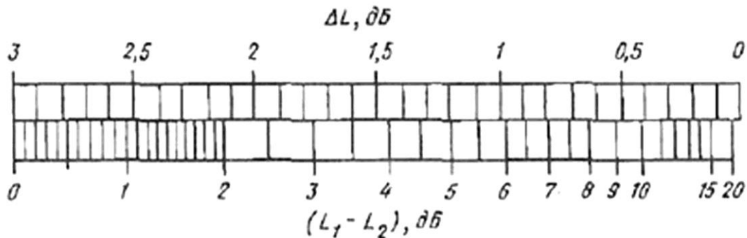
Рисунок 3.17 – Номограмма для логарифмического суммирования уровней звука
