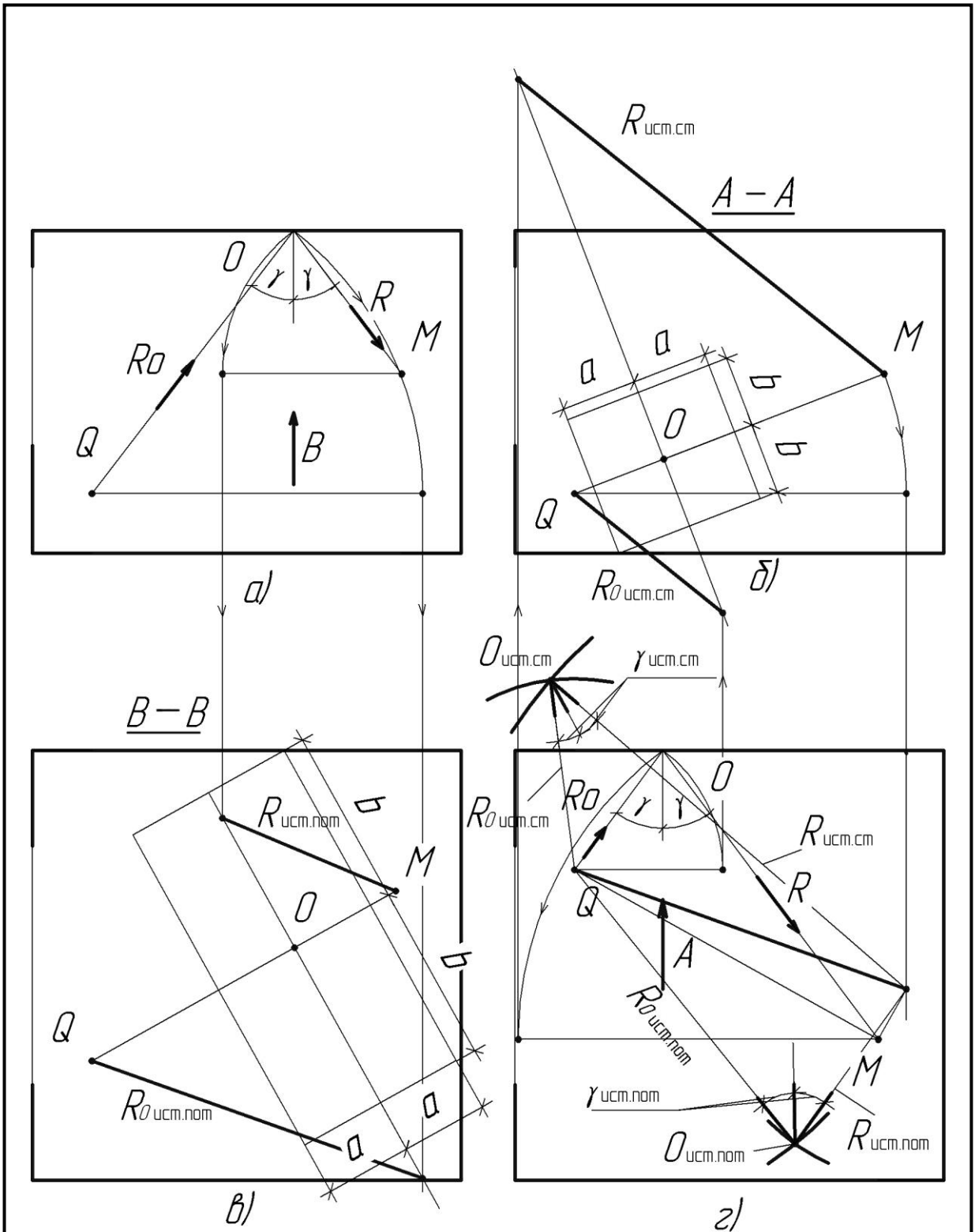
Рисунок 3.19 – Построение геометрических отражений (М 1:50)
