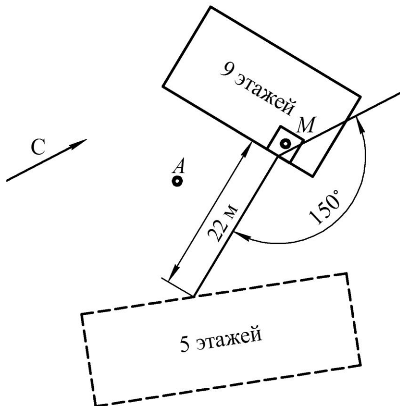
Рисунок 3.1 – Генплан к 1 разделу (М 1:500)
