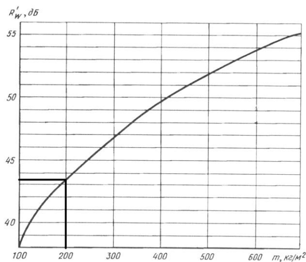
Рисунок 3.18 – Определение индекса изоляции воздушного шума
