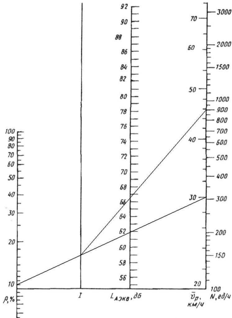
Рисунок 3.15 – Определение шумовой характеристики автомобильного транспорта
