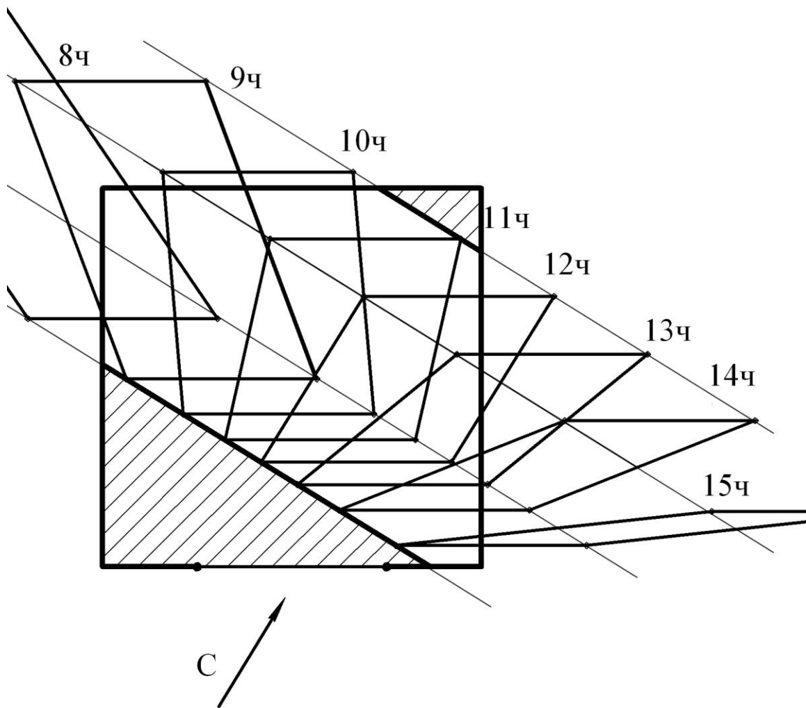
Рисунок 3.8 – Определение зоны инсоляции в помещении (М 1:50)
