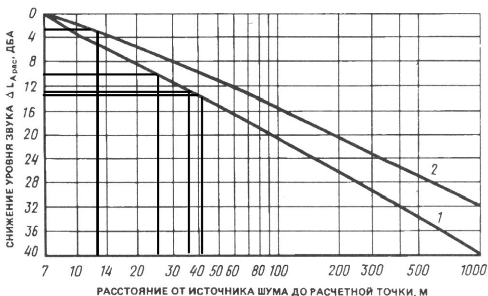
Рисунок 3.16 - Определение снижения уровня звука
